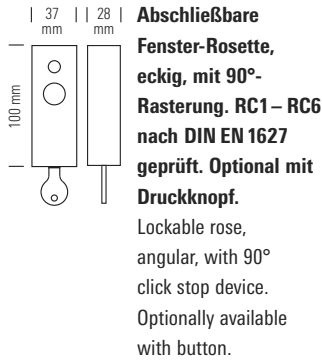
Abgerundete Fenster-Rosette mit 90°-Rasterung. Rounded window rose with 90° click stop device.
