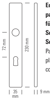
Abgerundetes Langschildpaar, blind. Pair of rounded long plates, blind.
