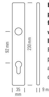
Eckiges Langschild- paar mit Bohrung für Profilzylinder, verdeckte Schraub- löcher.* Pair of angular long plates for euro stand- ard profile cylinder, concealed fixings.*
