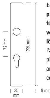
Eckiges Langschild- paar mit Bohrung für Buntbart- Schlüssel, verdeckte Schraublöcher.* Pair of angular long plates for standard key, concealed fixings.*
