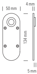
Abgerundetes Blind-Kurzschild- paar.* Pair of rounded blind short plates.*
